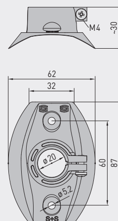
Plan coté (mm)
