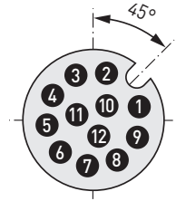
Разводка контактов (M12) AHT-30-AW
