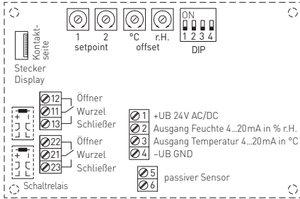
Schaltbild
