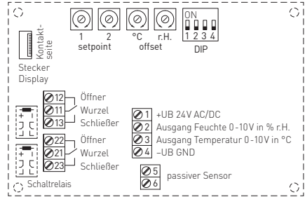
Schaltbild
