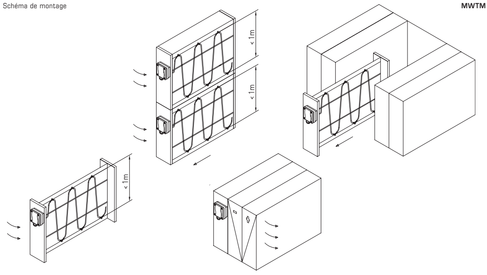
Schéma de montage
