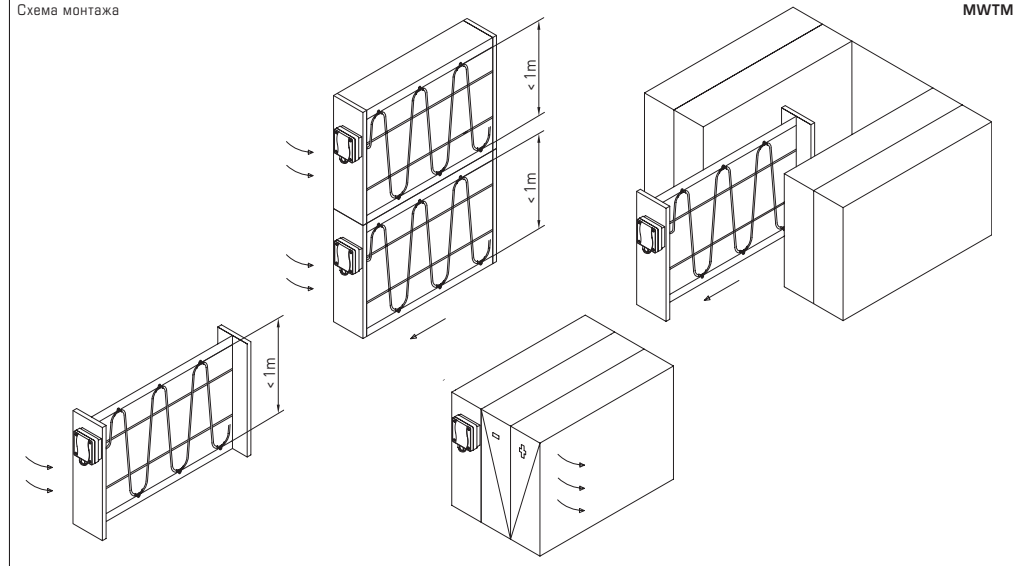
Схема монтажа
