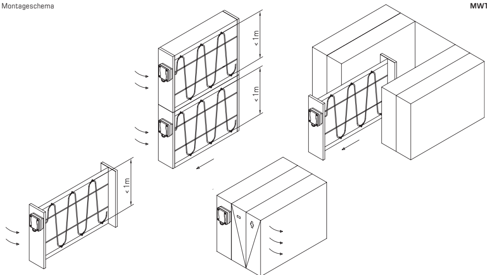
Montageschema
